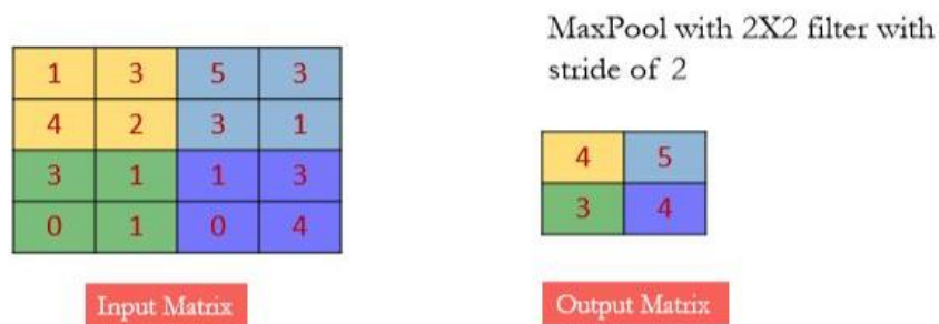
Figure 14. MaxPooling Layer
